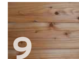
9 Nut- und Federbretter Breite: 146 mm Stärke: 19 mm
