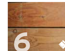
6 Rauschalung Breite: 150 mm Stärke: 24 mm
